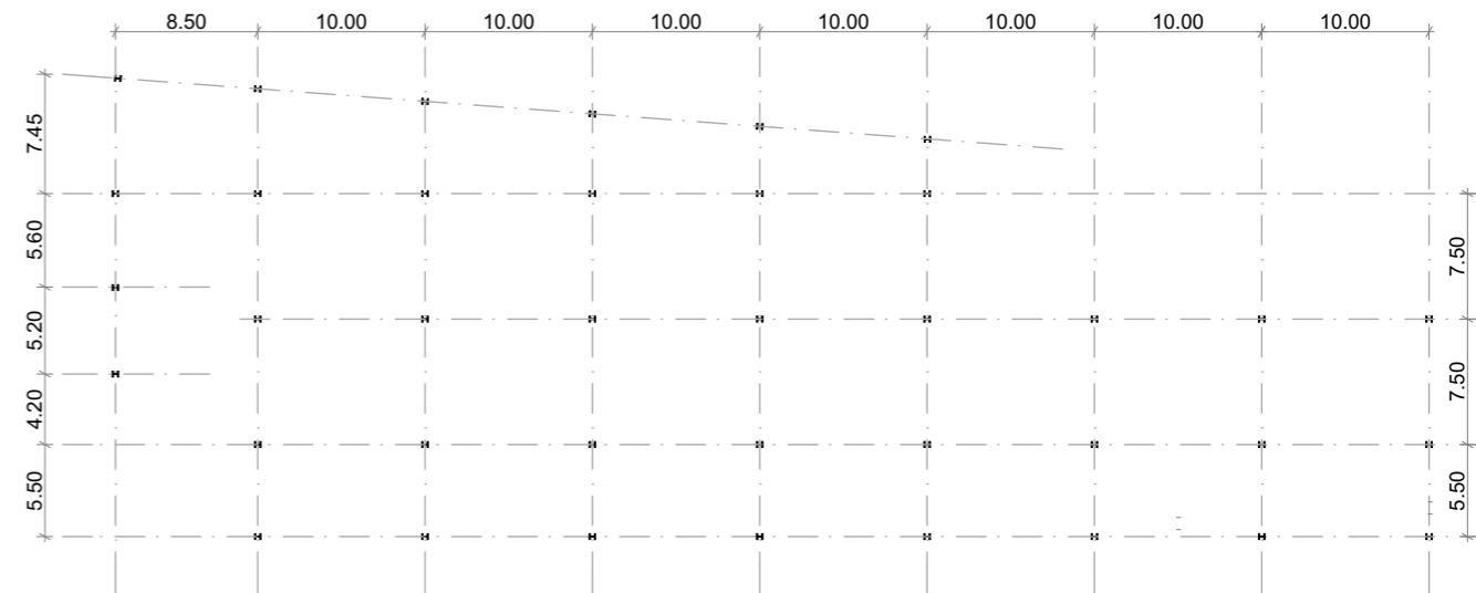
estrutura esc 1:500
